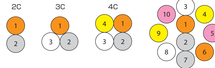
多対ケーブル/Multi pair cable
