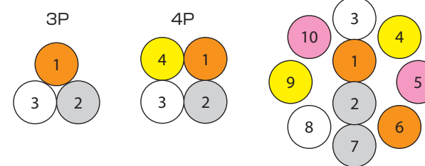
多対ケーブル/Multi pair cable
